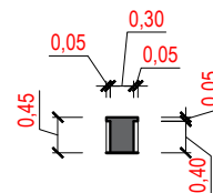
CORTE GG | BANCO 01 ESCALA 1/75
