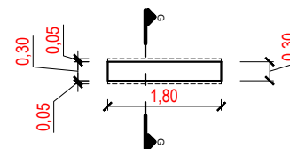
PLANTA BAIXA | BANCO 01 ESCALA 1/75
