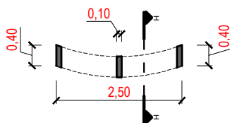
PLANTA BAIXA | BANCO 02 ESCALA 1/75
